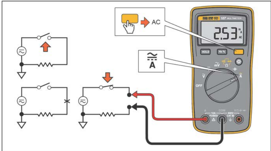
그림 3. AC 및 DC 전류 측정
