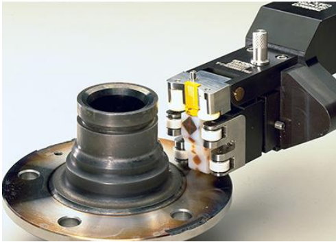
Spindle 크랙검사 (다중센서)
